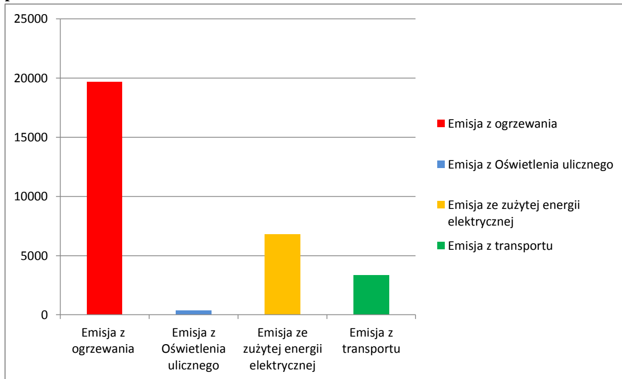
Rysunek 2. Emisja dwutlenku węgla (w Mg CO 2 ) w roku 2014 w podziale na źródła powstawania
