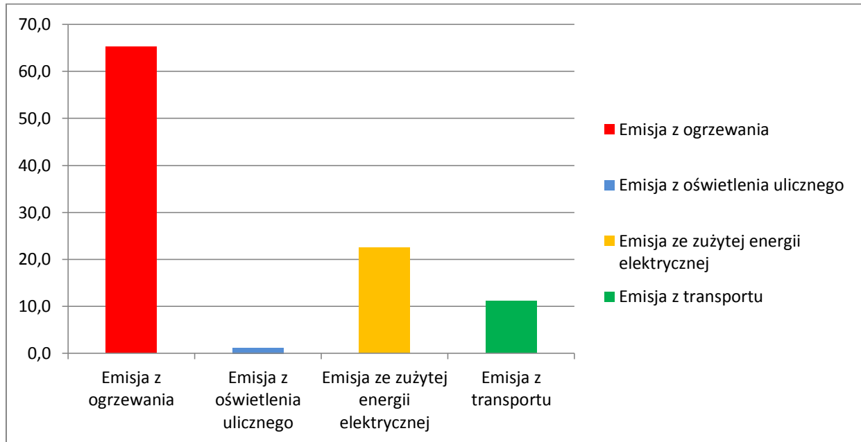
Rysunek 3. Procentowy udział emisji CO 2 z podziałem na źródła w 2014 roku
