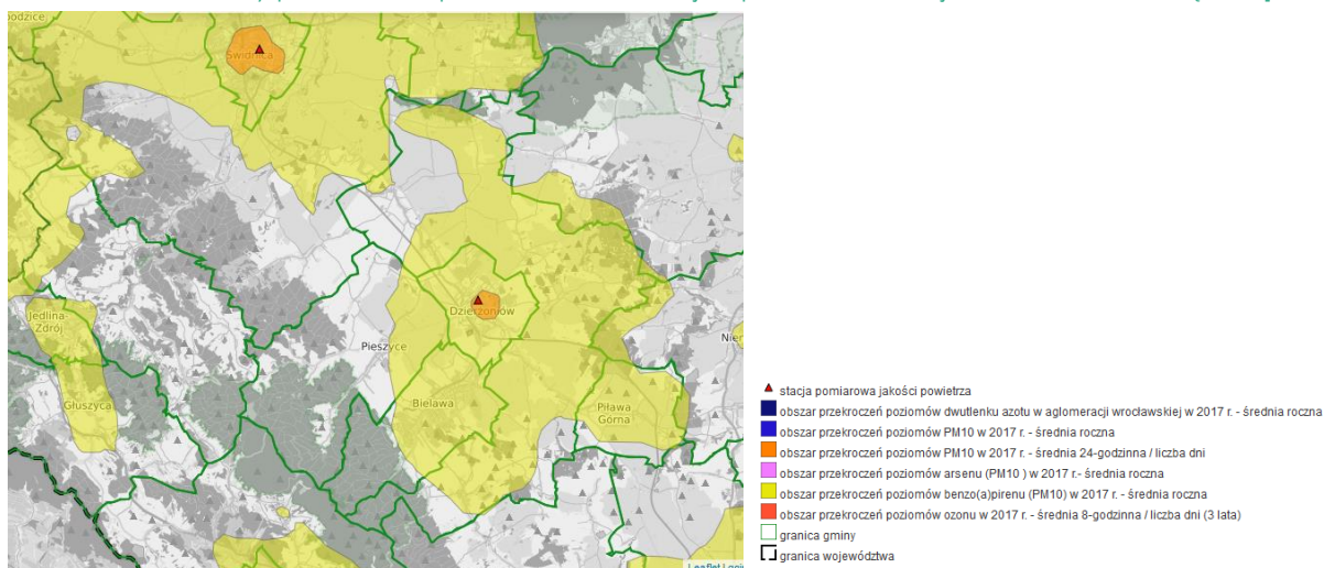
SCHEMAT 4. Obszary przekroczeń poziomów substancji w powietrzu w województwie dolnośląskim [2017].
